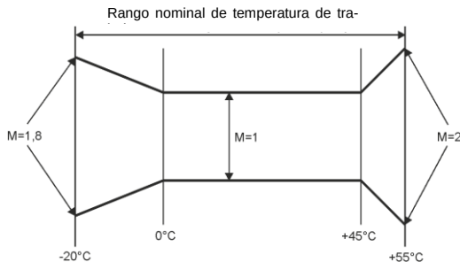
Fig. 42. El multiplicador de la incertidumbre básica dependiendo de la temperatura ambiente.
