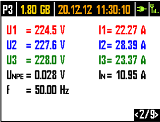
Fig. 6. Pantalla 2 con los valores eficaces de tensión y corriente.
