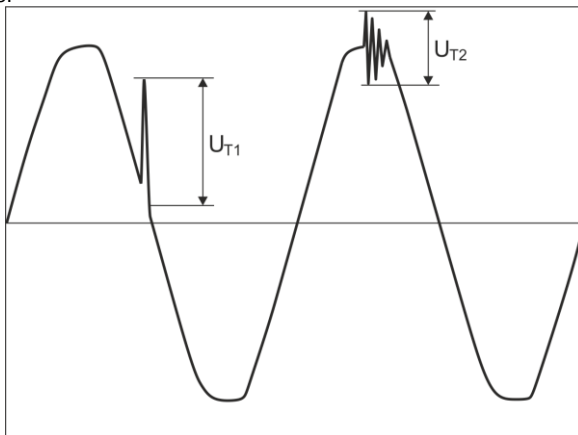
Fig. 41. Método para determinar las amplitudes de transientes.
