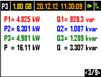
Fig. 7. Pantalla 3 con las potencias activas y reactivas.
