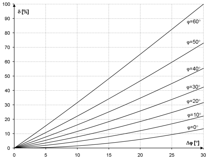
Fig. 43. La incertidumbre adicional resultante del error de fase, dependiendo del ángulo de desplazamiento de fase.
