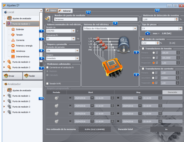
Fig. 27. Ajustes principales del punto de medición 1.
